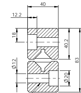
剖面 K-K
