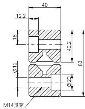
剖面 K-K
