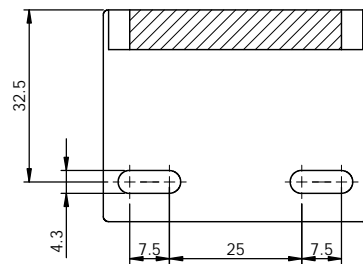
剖面 K-K
