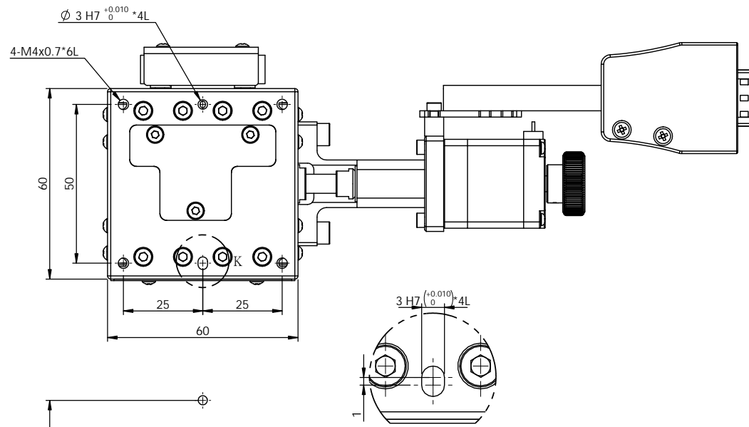
局部视图 K 比例 2:1
