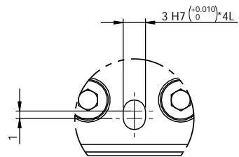
局部视图 K 比例 2:1
