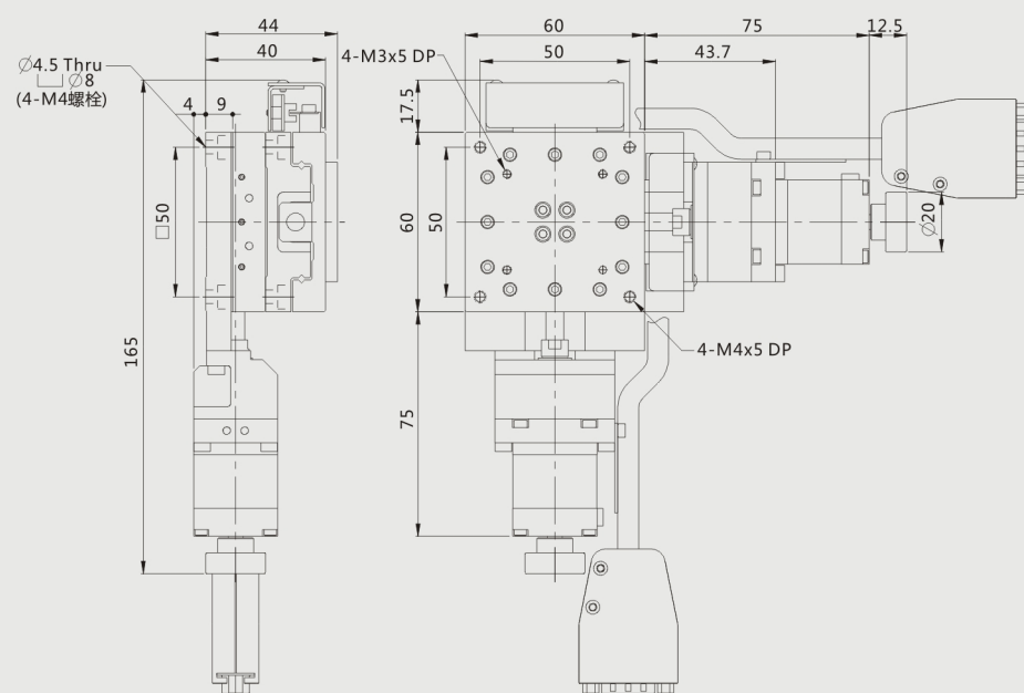
MXY60-A2N
