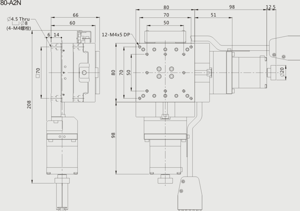
MXY80-A2N
